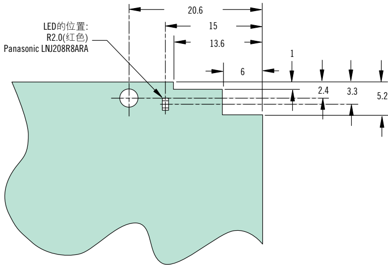
PCB板器件1面
