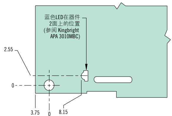
PCB板器件2面
