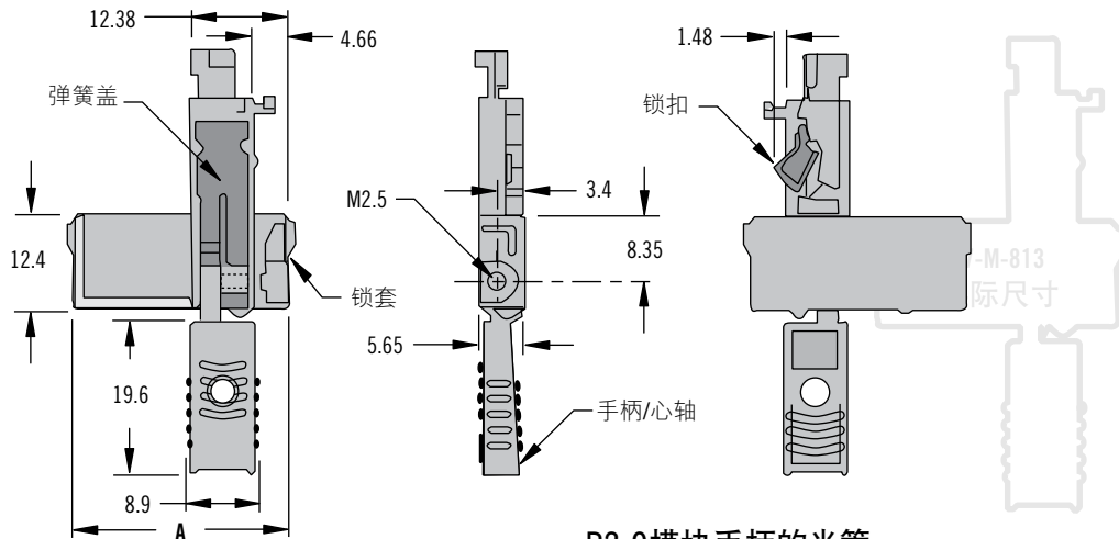
R2.0 模块手柄的光管
