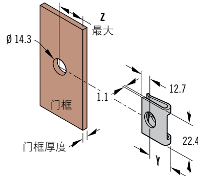
夹紧型搭扣
