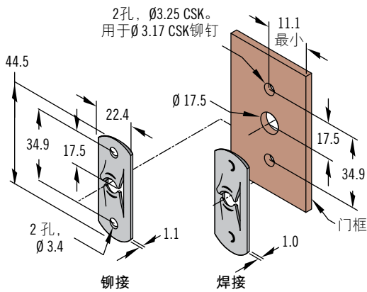
平片型搭扣
