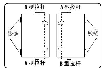
外视图
