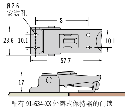
配有 91-634-XX 外露式保持器的门锁
