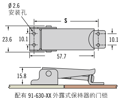
配有 91-630-XX 外露式保持器的门锁
